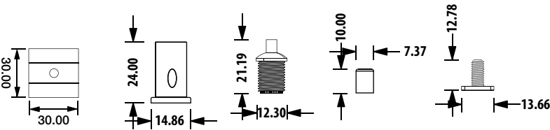
Pendant Accessories
